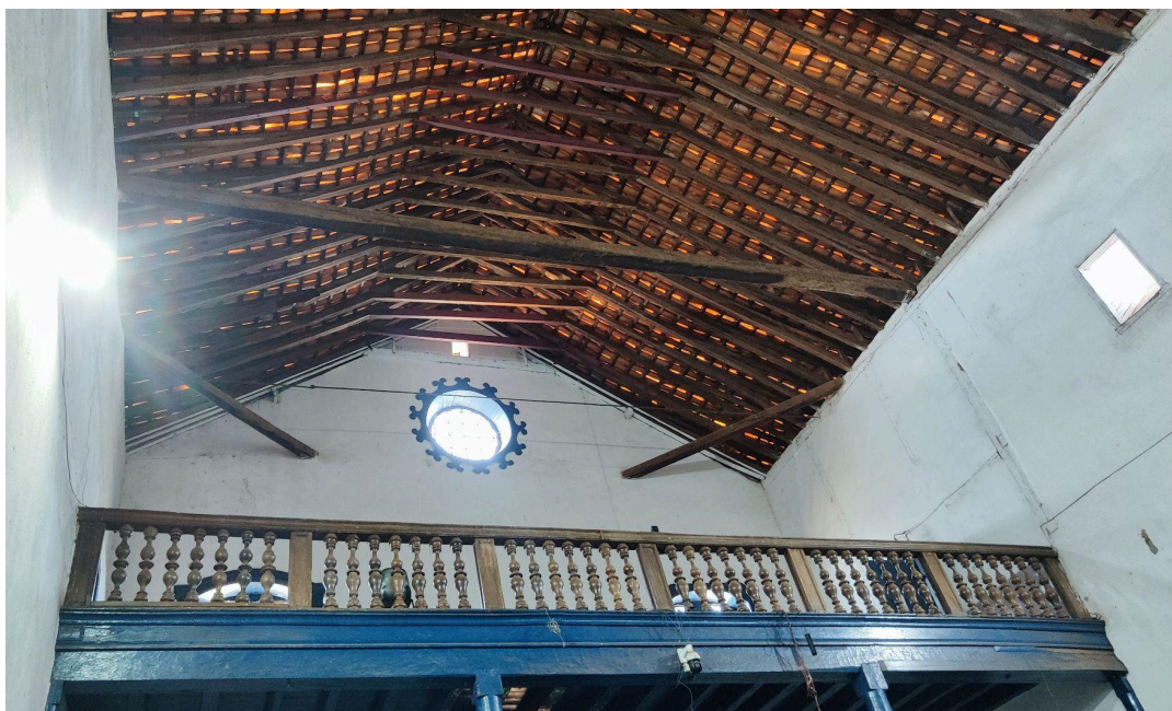
Reforço estrutural executado no telhado na nave Autoria: Francielle Ferreira Data: 06/05/2026
